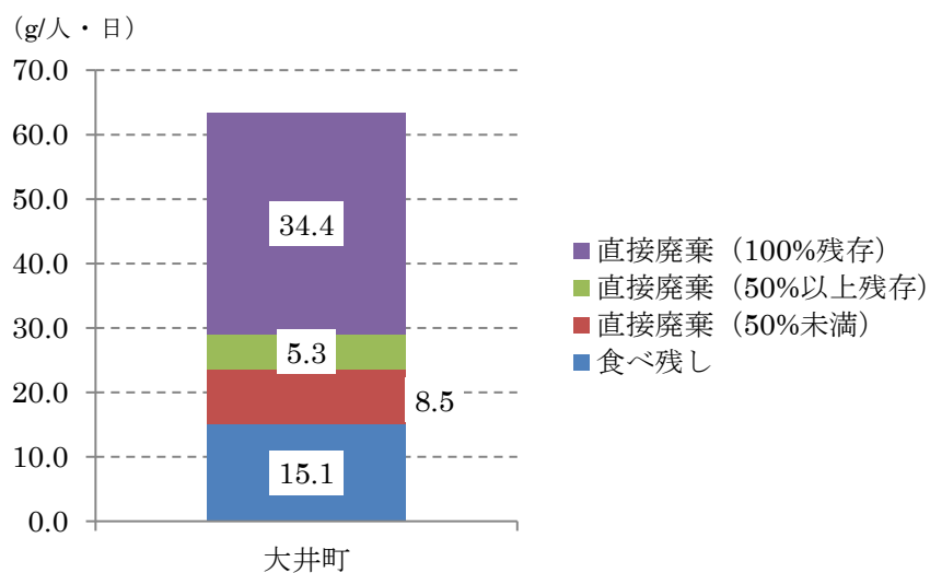
図表5 1人1日あたりの食品ロス発生量（大井町）
