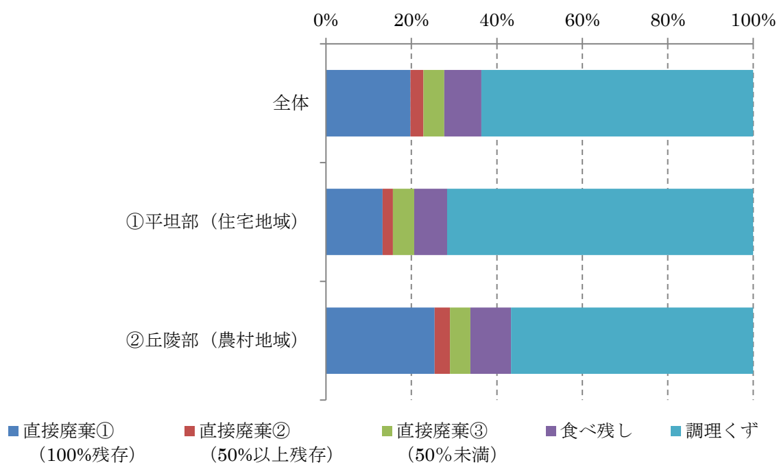
図表 4 食品ロス（直接廃棄、食べ残し）の割合（大井町）
