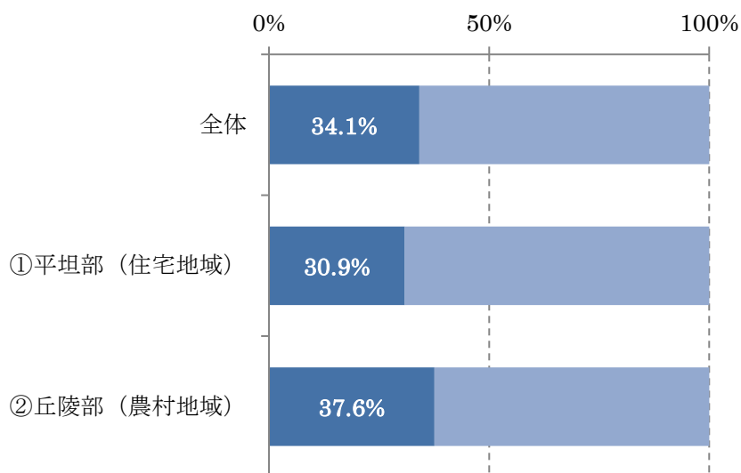
図表 3 試料中の食品廃棄物の割合（大井町）
