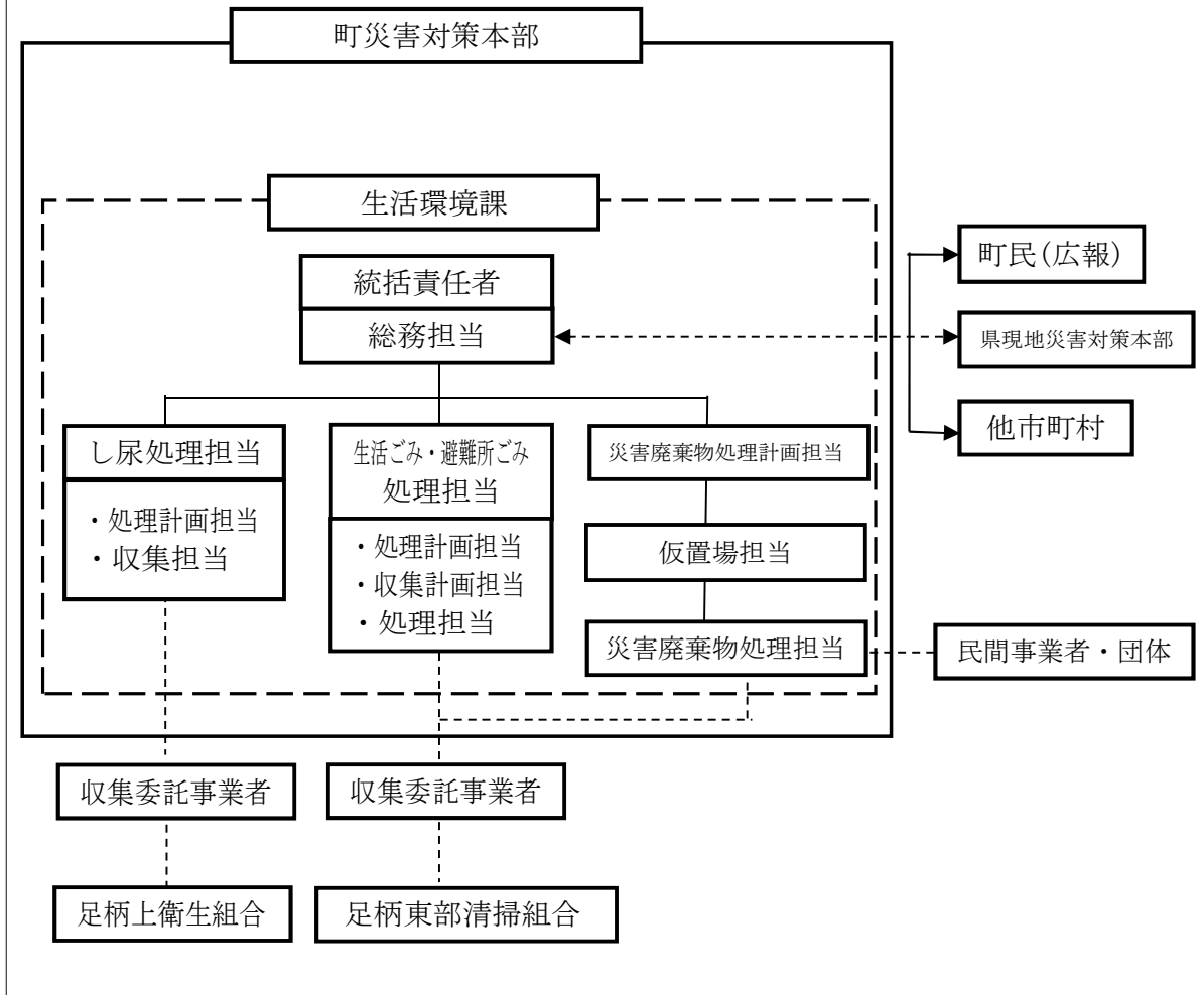
図1-3 災害対策本部が設置された場合の災害廃棄物処理体制の位置付け
