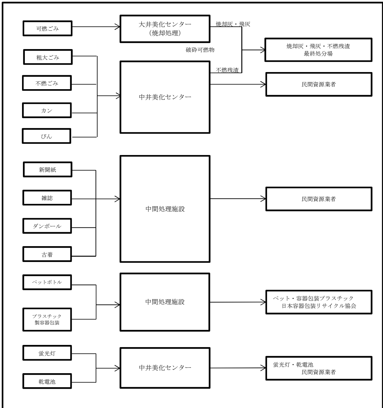
図3-3 ごみ処理フロー
