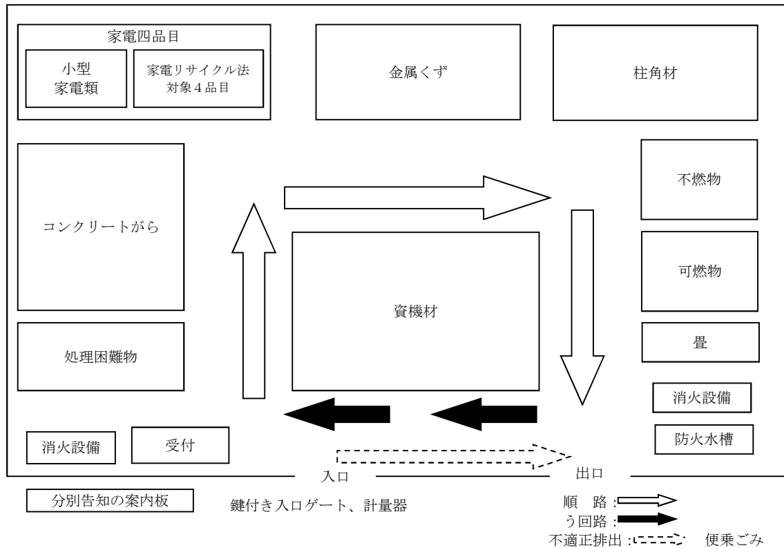
図3-7 一次仮置場レイアウト例
