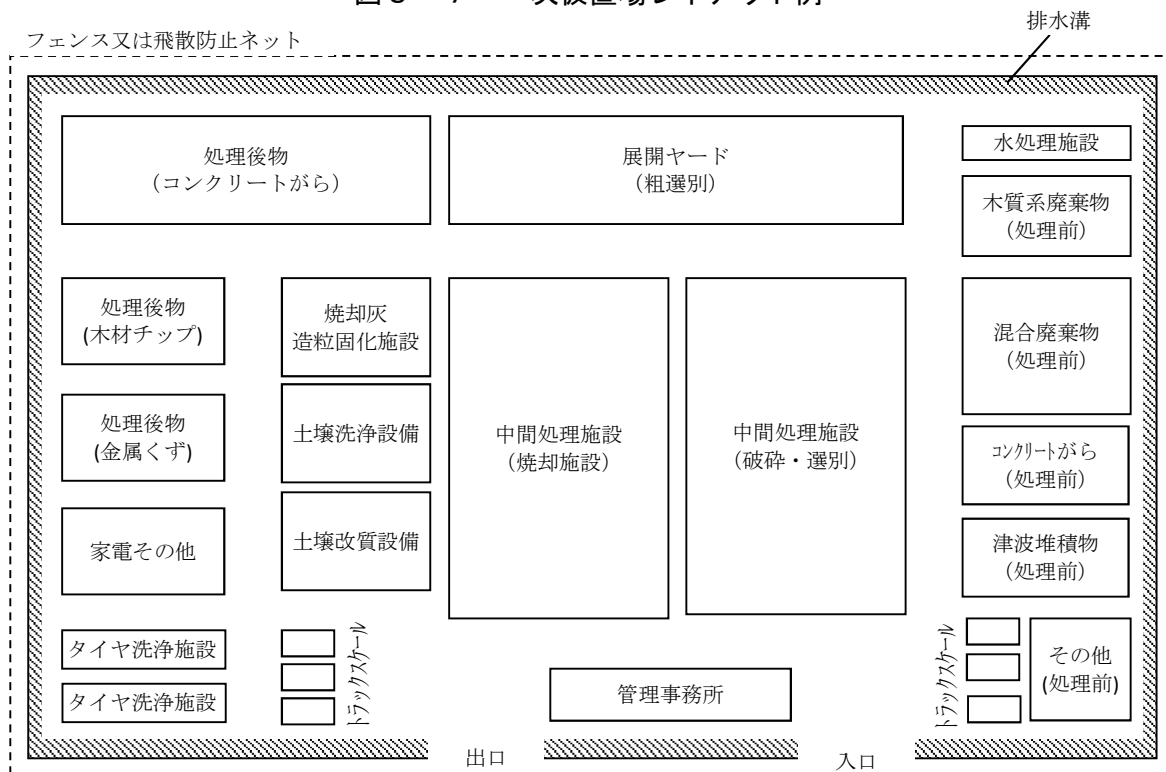
図3-7 一次仮置場レイアウト例
